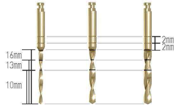
Ø1.3 Ø1.8 Ø2.3 DMD13 DMD18 DMD23
